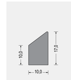
Part-Nr. 5830.5585 NR · grau VE: Bund á 100m
