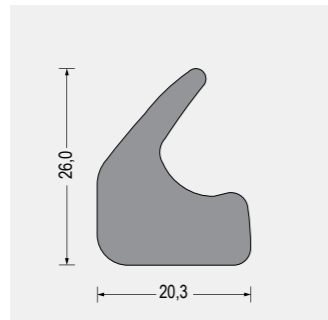
Part-Nr. 5800.5241 EPDM · grau VE: Bund á 25m
