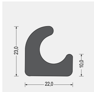
Part-Nr. 5800.8703 EPDM · schwarz VE: Bund á 25m
