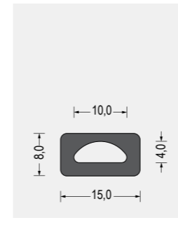
Part-Nr. 5800.4472 EPDM · schwarz VE: Bund á 100m
