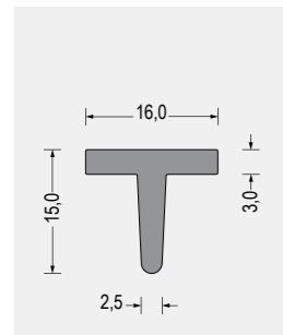
Part-Nr. 5800.7781 EPDM · grau VE: Bund á 25m
