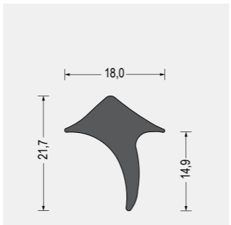
Part-Nr. 5800.6022 EPDM · schwarz VE: Bund á 50m
