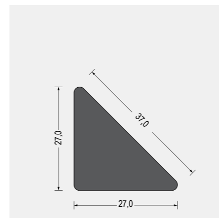
Part-Nr. 5800.5472 EPDM · schwarz VE: Bund á 25m
