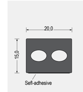
Part-Nr. 5880.5822 EPDM · schwarz VE: Bund á 25m als Montagehilfe einseitig selbstklebend
