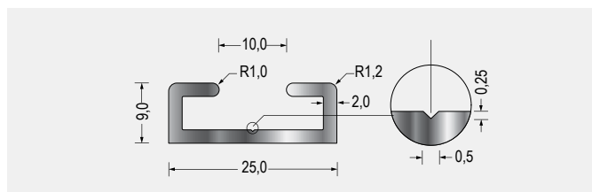
Part-Nr. 5400.3049 EPDM · 60° Shore A · schwarz VE: Lenght á 8m
