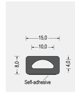
Part-Nr. 5880.4472 EPDM · schwarz VE: Bund á 100m als Montagehilfe einseitig selbstklebend
