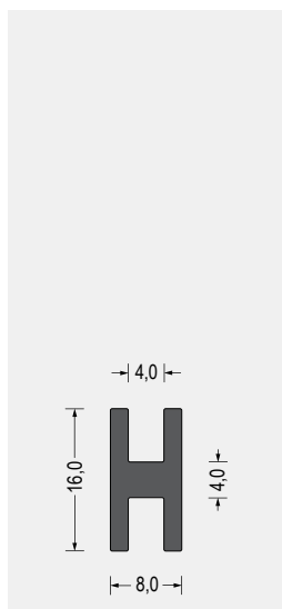
Part-Nr. 5400.2548 EPDM · 65° ShoreA schwarz VE: Bund á 50m
