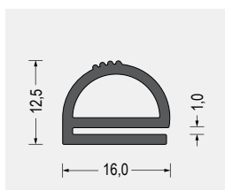
Part-Nr. 5500.1016 EPDM · 65° ShoreA · schwarz VE: Bund á 50m
