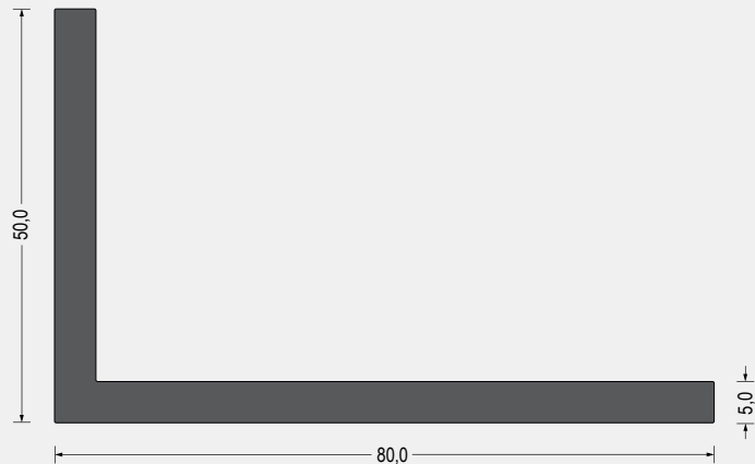
Part-Nr. 5400.1039 · EPDM · 70° ShoreA · schwarz · VE: Bund á 10m
