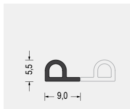
Part-Nr. 5400.5029 EPDM · 70° Shore A · schwarz VE: Spule á 200m Lieferform: 100 Doppelmeter mit Abrißkante
