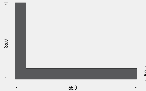
Part-Nr. 5400.1029 · EPDM · 68° ShoreA · schwarz · VE: Bund á 15m
