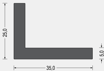
Part-Nr. 5400.1229 EPDM · 70° ShoreA · schwarz · VE: Bund á 25m
