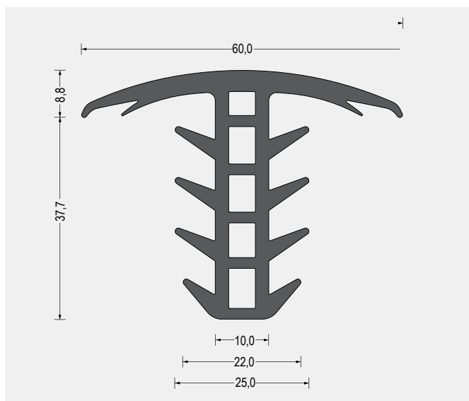
Part-Nr. 5400.3549 EPDM · 70° ShoreA · schwarz VE: Bund á 18m
