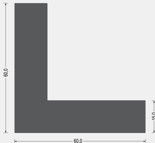
Part-Nr. 5400.1039 · EPDM · 70° ShoreA · schwarz · VE: Bund á 10m
