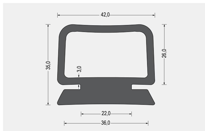
Part-Nr. 5400.3049 EPDM · 60° Shore A · schwarz VE: Lenght á 8m
