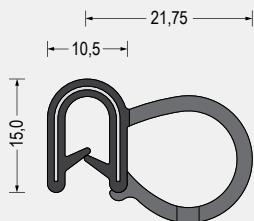
Part-Nr. 5610.4249 EPDM-Weichgummi/ EPDM-Moosgummi · schwarz Klemmbereich 1-3,5mm VE: Bund á 50m
