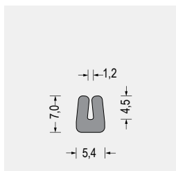
Part-Nr. 8800.7652 EPDM · grau VE: Bund á 100m
