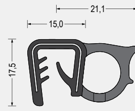
Part-Nr. 5610.4259 EPDM-Weichgummi/ EPDM-Moosgummi · schwarz Klemmbereich 5-9mm VE: Bund á 50m
