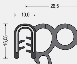
Part-Nr. 5610.6309 EPDM-Weichgummi/ EPDM-Moosgummi · schwarz Klemmbereich 1,5-3,5mm VE: Bund á 25m
