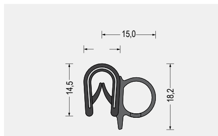
Part-Nr. 5610.2469 Weich-PVC/EPDM-Moosgummi · schwarz Klemmbereich 1-4mm VE: Bund á 50m
