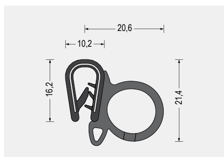
Part-Nr. 5610.2325 Weich-PVC/EPDM-Moosgummi · schwarz Klemmbereich 1-2,5mm VE: Bund á 50m
