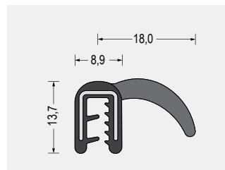
Part-Nr. 5610.4269 EPDM-Weichgummi/ EPDM-Moosgummi · schwarz Klemmbereich 2-3mm VE: Bund á 50m
