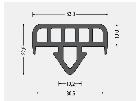
Part-Nr. 5400.4510 EPDM · 70° ShoreA · schwarz VE: Bund á 25m
