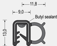
Part-Nr. 5610.6207 EPDM-Weichgummi/ EPDM-Moosgummi · schwarz mit eingespritzter Butylschnur Klemmbereich 2mm VE: Bund á 50m
