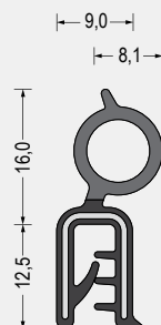
Part-Nr. 5610.6259 EPDM-Weichgummi/ EPDM-Moosgummi · schwarz Klemmbereich 1-2,5mm VE: Bund á 100m
