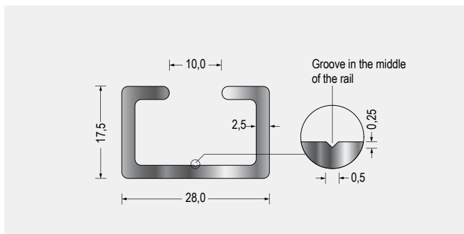
Part-Nr. 5150.7080 Halteleiste für Polsterprofile (nicht geeignet für Profil 547.4356) Aluminium blank VE: Lenght á 5m · Mindestmenge 10m
