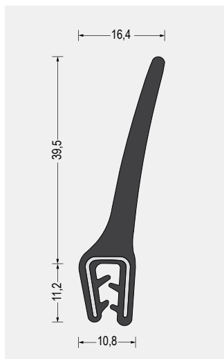
Part-Nr. 5610.3269 EPDM-Weichgummi · schwarz Klemmbereich 2-4mm VE: Bund á 25m
