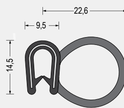
Part-Nr. 5610.4284 EPDM-Weichgummi/ EPDM-Moosgummi · schwarz Klemmbereich 1,5-3mm VE: Bund á 50m
