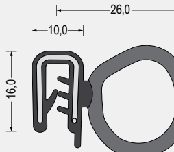
Part-Nr. 5610.4291 EPDM-Weichgummi/ EPDM-Moosgummi · schwarz Klemmbereich 1-3,5mm VE: Bund á 50m
