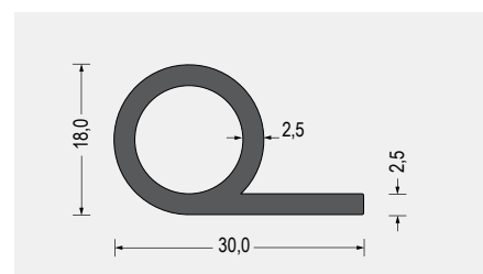
Part-Nr. 5400.5188 EPDM · 68° ShoreA · schwarz VE: Bund á 25m
