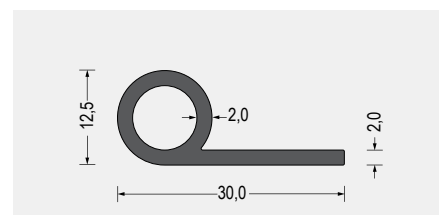
Part-Nr. 5400.5127 EPDM · 70° ShoreA · schwarz VE: Bund á 50m
