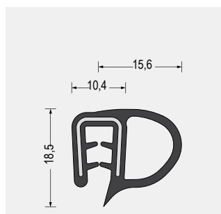
Part-Nr. 5640.6309 Silikon · schwarz Klemmbereich 2,5-4,5mm VE: Bund á 25m
