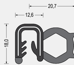
Part-Nr. 5610.4499 EPDM-Weichgummi/ EPDM-Moosgummi · schwarz Klemmbereich 3-5mm VE: Bund á 50m
