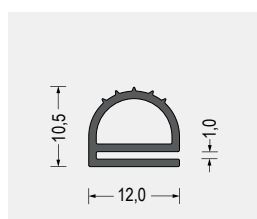
Part-Nr. 5500.1012 EPDM · 65° ShoreA · schwarz VE: Bund á 50m
