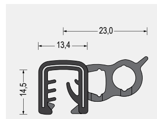
Part-Nr. 5610.6399 EPDM-Weichgummi/ EPDM-Moosgummi · schwarz Klemmbereich 5-6mm VE: Bund á 50m
