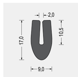
Part-Nr. 5800.6372 EPDM · schwarz VE: Bund á 50m
