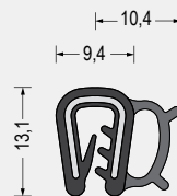
Part-Nr. 5610.6219 EPDM-Weichgummi/ EPDM-Moosgummi · schwarz Klemmbereich 2mm VE: Bund á 50m
