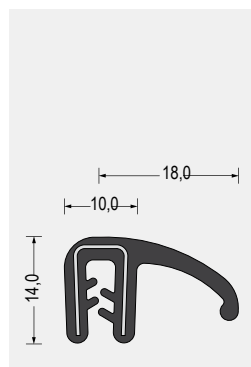
Part-Nr. 5640.3449 Silikon · schwarz Klemmbereich 1-3mm VE: Bund á 25m
