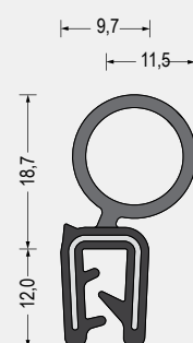
Part-Nr. 5610.6409 EPDM-Weichgummi/ EPDM-Moosgummi · schwarz Klemmbereich 1-3mm VE: Bund á 50m
