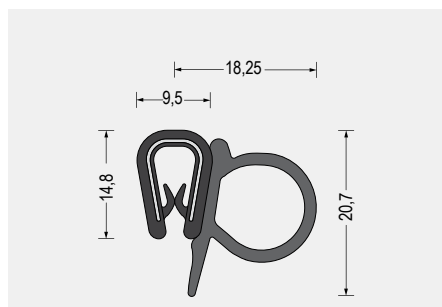
Part-Nr. 5610.2869 Weich-PVC/EPDM-Moosgummi · schwarz Klemmbereich 1-4mm VE: Bund á 50m
