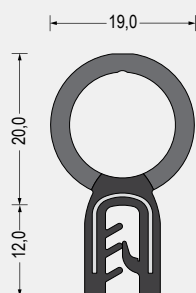
Part-Nr. 5610.6389 EPDM-Weichgummi/ EPDM-Moosgummi · schwarz Klemmbereich 1-2mm VE: Bund á 50m
