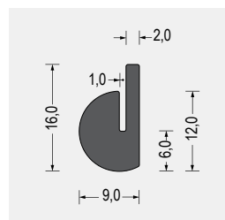
Part-Nr. 5800.5082 EPDM · schwarz VE: Bund á 50m
