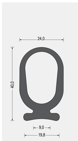
Part-Nr. 5400.3139 EPDM · 70° Shore A · schwarz VE: Bund á 25m
