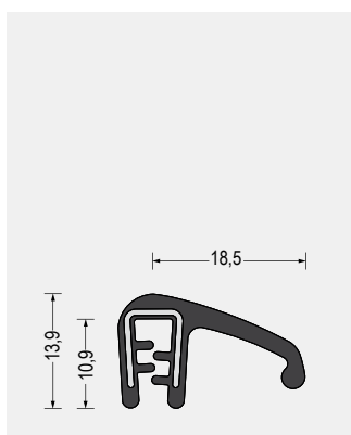
Part-Nr. 5610.3449 EPDM-Weichgummi · schwarz Klemmbereich 1-3mm VE: Bund á 50m
