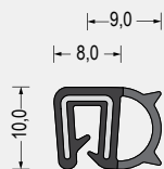
Part-Nr. 5610.6699 EPDM-Weichgummi/ EPDM-Moosgummi · schwarz Klemmbereich 1-2,5mm VE: Bund á 100m
