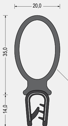
Part-Nr. 5610.2001 Weich-PVC/EPDM-Weichgummi schwarz Klemmbereich 2-4mm VE: Bund á 25m
