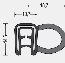
Part-Nr. 5610.8559 EPDM-Weichgummi/ EPDM-Moosgummi · schwarz Brandschutzqualität nach EN 45545 Klemmbereich 1,5-3mm VE: Bund á 25m
