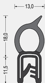
Part-Nr. 5610.6268 EPDM-Weichgummi/ EPDM-Moosgummi · schwarz Klemmbereich 2-4mm VE: Bund á 50m
