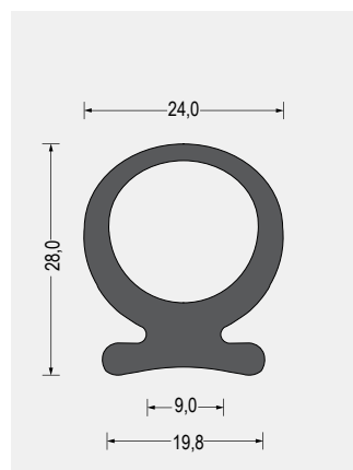
Part-Nr. 5400.3129 EPDM · 70° Shore A · schwarz VE: Bund á 30m
