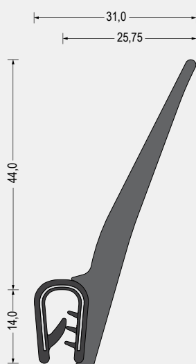
Part-Nr. 5610.2529 Weich-PVC/EPDM-Moosgummi · schwarz Klemmbereich 2,5-4mm VE: Bund á 25m
