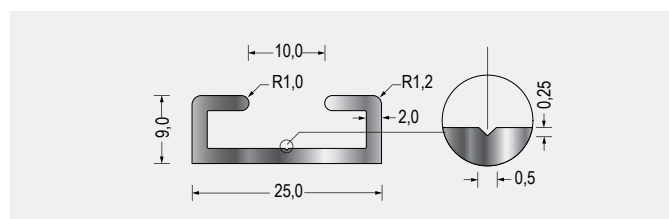
Part-Nr. 5150.5010 Halteleiste für Rolltorprofile, Aluminium blank nicht oder nur sehr bedingt geeignet für Profile: 5430.3019 / 5400.3029 / 5400.3079 / 5400.3049 VE: Lenght á 5m, Mindestmenge 10m
