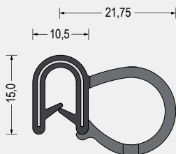
Part-Nr. 5610.4245 CR-Weichgummi/ CR-Moosgummi · schwarz Klemmbereich 1-3,5mm VE: Bund á 25m
