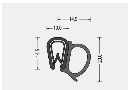
Part-Nr. 5610.2022 Weich-PVC/EPDM-Moosgummi · schwarz Klemmbereich 1-4mm VE: Bund á 50m
