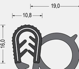
Part-Nr. 5610.5599 EPDM-Weichgummi/ EPDM-Moosgummi · schwarz Klemmbereich 2-4mm VE: Bund á 25m
