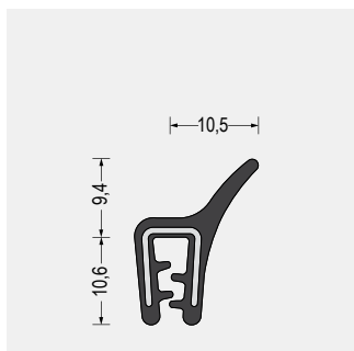
Part-Nr. 5610.3329 EPDM-Weichgummi · schwarz Klemmbereich 1-3mm VE: Bund á 50m
