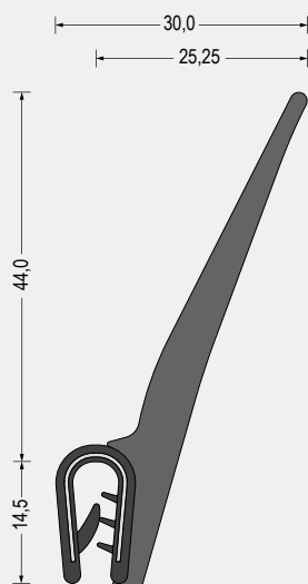
Part-Nr. 5610.2527 Weich-PVC/EPDM-Moosgummi · schwarz Klemmbereich 1-2,5mm VE: Bund á 25m
