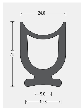
Part-Nr. 5400.3169 EPDM · 70° Shore A · schwarz VE: Bund á 25m
