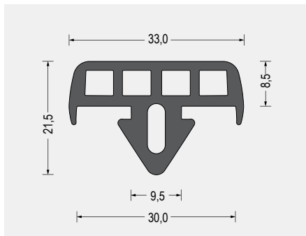
Part-Nr. 5400.4409 EPDM · 70° ShoreA · schwarz VE: Bund á 25m
