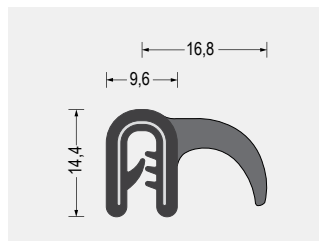
Part-Nr. 5610.4229 EPDM-Weichgummi/ EPDM-Moosgummi · schwarz Klemmbereich 1-2,5mm VE: Bund á 100m
