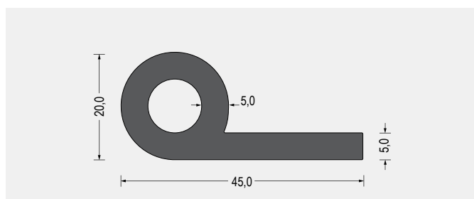
Part-Nr. 5410.5201 CR · 70° ShoreA · schwarz VE: Bund á 25m
