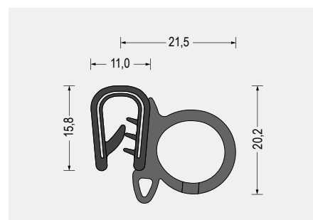
Part-Nr. 5610.2327 Weich-PVC/EPDM-Moosgummi · schwarz Klemmbereich 4-6mm VE: Bund á 50m
