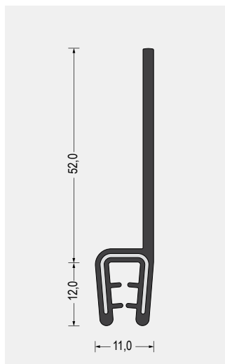
Part-Nr. 5610.3229 EPDM-Weichgummi · schwarz Klemmbereich 3-4mm VE: 40m (2 Lengthn á 20m)
