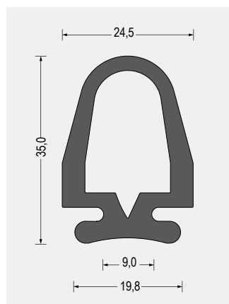
Part-Nr. 5400.3159 EPDM · 70° Shore A · schwarz VE: Bund á 30m
