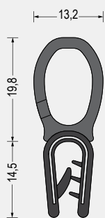
Part-Nr. 5610.2517 Weich-PVC/EPDM-Moosgummi schwarz Klemmbereich 1-2,5mm VE: Bund á 50m
