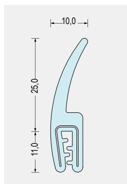
Part-Nr. 5640.3320 Silikon · transparent mit Edelstahlband Klemmbereich 1-2,5mm VE: Bund á 50m
