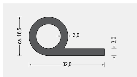
Part-Nr. 5400.5161 EPDM · 65° ShoreA · schwarz VE: Bund á 50m
