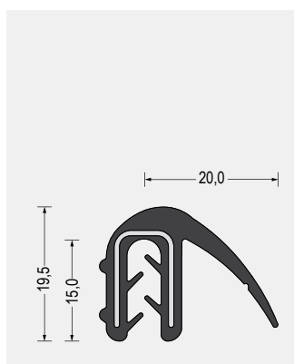
Part-Nr. 5610.3339 EPDM-Weichgummi · schwarz Klemmbereich 1-3,5mm VE: Bund á 25m
