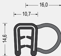
Part-Nr. 5610.6289 EPDM-Weichgummi/ EPDM-Moosgummi · schwarz Klemmbereich 1,5-3mm VE: Bund á 50m
