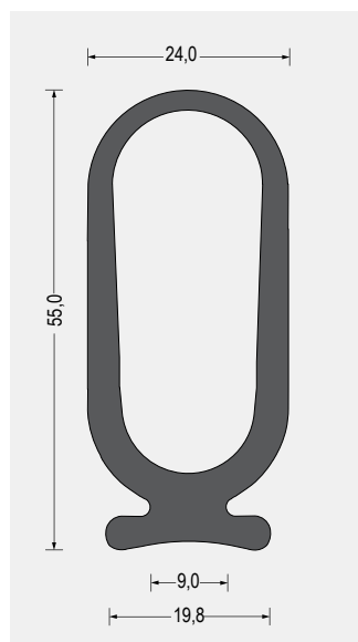
Part-Nr. 5400.3149 EPDM · 70° Shore A · schwarz VE: Bund á 15m
