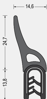
Part-Nr. 5610.2539 Weich-PVC/EPDM-Moosgummi schwarz Klemmbereich 1,5-3,5mm VE: Bund á 50m
