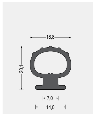
Part-Nr. 5400.3029 EPDM · 70° Shore A · schwarz VE: Bund á 25m
