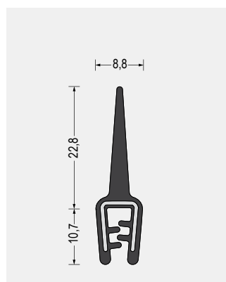
Part-Nr. 5610.3249 EPDM-Weichgummi · schwarz Klemmbereich 1-3mm VE: Bund á 50m
