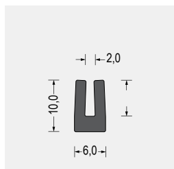
Part-Nr. 5800.6582 EPDM · schwarz VE: Bund á 100m
