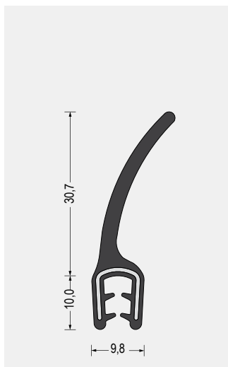
Part-Nr. 5610.3259 EPDM-Weichgummi · schwarz Klemmbereich 2-4mm VE: Bund á 50m
