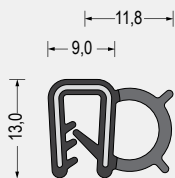
Part-Nr. 5610.8209 EPDM-Weichgummi/ EPDM-Moosgummi · schwarz Brandschutzqualität nach EN 45545 Klemmbereich 2mm VE: Bund á 50m
