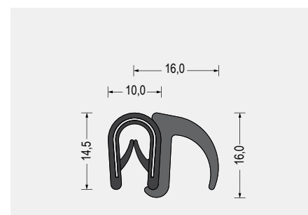
Part-Nr. 5610.2449 Weich-PVC/EPDM-Moosgummi · schwarz Klemmbereich 1-4mm VE: Bund á 50m
