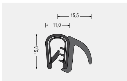
Part-Nr. 5610.2485 Weich-PVC/EPDM-Moosgummi · schwarz Klemmbereich 4-6mm VE: Bund á 50m
