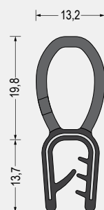
Part-Nr. 5610.6375 NBR-Weichgummi/ NBR-Moosgummi · schwarz Klemmbereich 3-5mm VE: Bund á 50m
