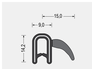
Part-Nr. 5610.4214 EPDM-Weichgummi/ EPDM-Moosgummi · schwarz Klemmbereich 1-3mm VE: Bund á 50m
