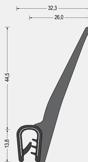
Part-Nr. 5610.2528 Weich-PVC/EPDM-Moosgummi · schwarz Klemmbereich 4-6mm VE: Bund á 25m
