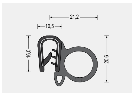
Part-Nr. 5610.2326 Weich-PVC/EPDM-Moosgummi · schwarz Klemmbereich 2,5-4mm VE: Bund á 50m
