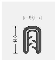
Part-Nr. 5610.1999 Weich-PVC · schwarz Klemmbereich 1-2,5mm VE: Bund á 50m
