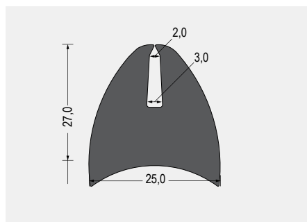
Part-Nr. 5500.0298 EPDM · 55° ShoreA · schwarz VE: Bund á 25m
