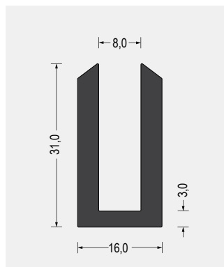
Part-Nr. 5500.0801 EPDM · 70° ShoreA · schwarz VE: Bund á 25m
