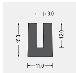
Part-Nr. 5800.5862 EPDM · schwarz VE: Bund á 50m
