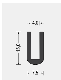
Part-Nr. 5500.0464 EPDM · 60° ShoreA schwarz VE: Bund á 100m
