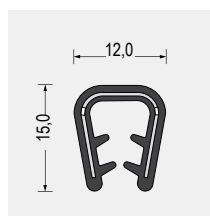
Part-Nr. 5610.0819 Soft Rubber EPDM schwarz Klemmbereich 3-6mm VE: Bund á 100m
