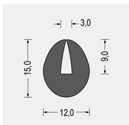
Part-Nr. 5800.7392 EPDM · schwarz VE: Bund á 50m
