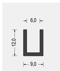
Part-Nr. 5500.0602 EPDM · 65° ShoreA schwarz VE: Bund á 100m
