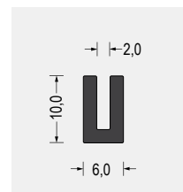
Part-Nr. 5500.0211 EPDM · 70° ShoreA schwarz VE: Bund á 100m
