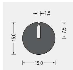
Part-Nr. 5800.9153 EPDM · schwarz VE: Bund á 50m
