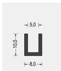
Part-Nr. 5500.0508 EPDM · 65° ShoreA schwarz VE: Bund á 100m
