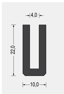
Part-Nr. 5510.0405 CR · 60° ShoreA schwarz VE: Bund á 25m
