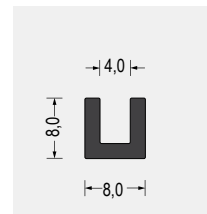
Part-Nr. 5500.0418 EPDM · 65° ShoreA schwarz VE: Bund á 100m
