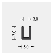
Part-Nr. 5500.0316 EPDM · 65° ShoreA schwarz VE: Bund á 100m
