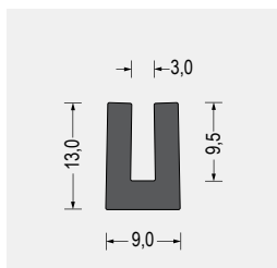
Part-Nr. 5800.5962 EPDM · schwarz VE: Bund á 50m
