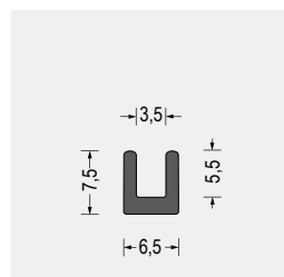
Part-Nr. 5800.6935 EPDM · schwarz VE: Bund á 100m
