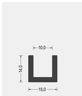
Part-Nr. 5500.1009 EPDM · 65° ShoreA · schwarz VE: Bund á 50m
