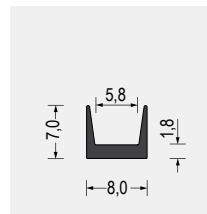
Part-Nr. 5500.0607 EPDM · 70° ShoreA schwarz VE: Bund á 100m
