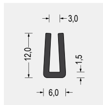
Part-Nr. 5500.0318 EPDM · 60° ShoreA schwarz VE: Bunde á 100m
