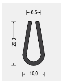
Part-Nr. 5500.0703 EPDM · 60° ShoreA schwarz VE: Bund á 50m
