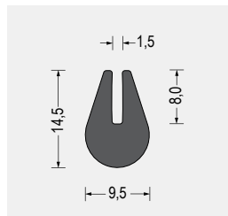
Part-Nr. 5800.8862 EPDM · schwarz VE: Bund á 50m
