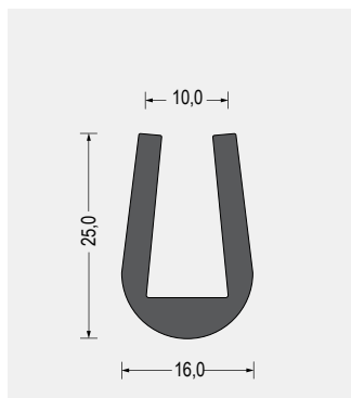
Part-Nr. 5500.1002 EPDM · 45° ShoreA · schwarz VE: Bund á 50m
