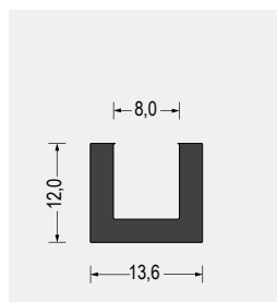
Part-Nr. 5510.0804 CR · 60° ShoreA schwarz VE: Bund á 40m
