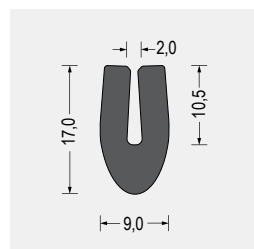
Part-Nr. 5800.6372 EPDM · schwarz VE: Bund á 50m
