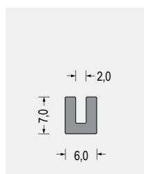
Part-Nr. 5540.0248 60° ShoreA · grau VE: Bund á 50m
