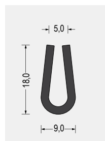
Part-Nr. 5500.0503 EPDM · 65° ShoreA schwarz VE: Bund á 100m
