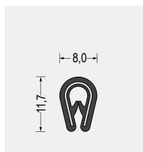
Part-Nr. 5610.1408 Weich-PVC · schwarz Klemmbereich 1-2,5mm VE: Bund á 100m
