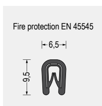
Part-Nr. 5610.8119 Soft Rubber EPDM schwarz Brandschutzqualität EN 45545 Klemmbereich 1-2mm VE: Bund á 100m
