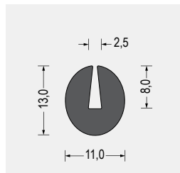
Part-Nr. 5800.8052 EPDM · schwarz VE: Bund á 50m
