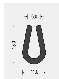
Part-Nr. 5500.0601 EPDM · 60° ShoreA schwarz VE: Bund á 100m
