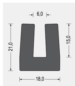
Part-Nr. 5800.7371 EPDM · schwarz VE: Bund á 50m
