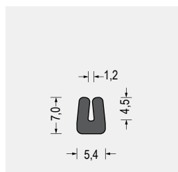
Part-Nr. 5800.7652 EPDM · schwarz VE: Bund á 200m
