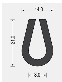
Part-Nr. 5500.0815 EPDM · 70° ShoreA schwarz VE: Bund á 40m
