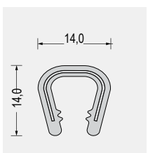
Part-Nr. 5610.1913 Weich-PVC · hellgrau Klemmbereich 8-10mm VE: Bund á 100m
