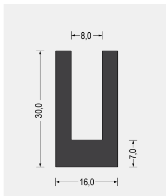
Part-Nr. 5500.0802 EPDM · 65° ShoreA · schwarz VE: Bund á 25m
