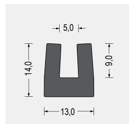
Part-Nr. 5800.5052 EPDM · schwarz VE: Bund á 50m
