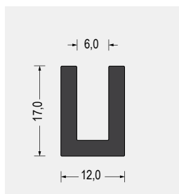
Part-Nr. 5500.0606 EPDM · 70° ShoreA schwarz VE: Bund á 50m
