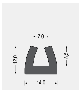
Part-Nr. 5800.7077 EPDM · schwarz VE: Bund á 50m
