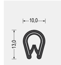
Part-Nr. 5610.1469 Weich-PVC · schwarz Klemmbereich 1-4mm VE: Bund á 100m
