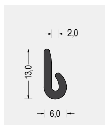
Part-Nr. 5500.0204 EPDM · 65° ShoreA schwarz VE: Bund á 100m
