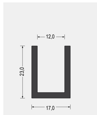
Part-Nr. 5500.1204 EPDM · 70° ShoreA · schwarz VE: Bund á 50m
