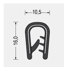
Part-Nr. 5610.1439 Weich-PVC · schwarz Klemmbereich 2-4mm VE: Bund á 100m
