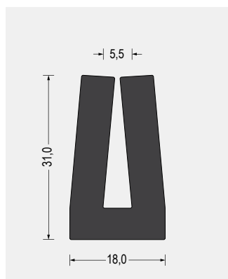
Part-Nr. 5500.0593 EPDM · 70° ShoreA · schwarz VE: Bund á 15m rundgeheizt, talkumiert
