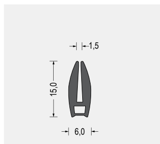
Part-Nr. 5500.0177 EPDM · 65° ShoreA · schwarz VE: Bund á 100m
