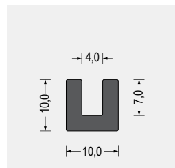
Part-Nr. 5800.4011 EPDM · schwarz VE: Bund á 50m
