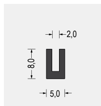
Part-Nr. 5500.0205 EPDM · 60° ShoreA schwarz VE: Bund á 100m
