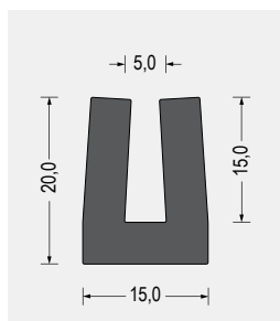
Part-Nr. 5800.7792 EPDM · schwarz VE: Bund á 25m
