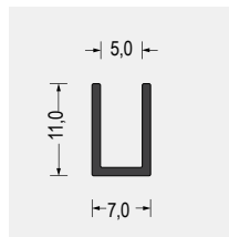
Part-Nr. 5500.0566 EPDM · 65° ShoreA schwarz VE: Bund á 100m
