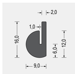
Part-Nr. 5800.5082 EPDM · schwarz VE: Bund á 50m
