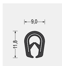
Part-Nr. 5610.1309 Weich-PVC · schwarz Klemmbereich 1-3mm VE: Bund á 100m
