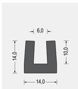
Part-Nr. 5820.6122 NBR · schwarz VE: Bund á 50m
