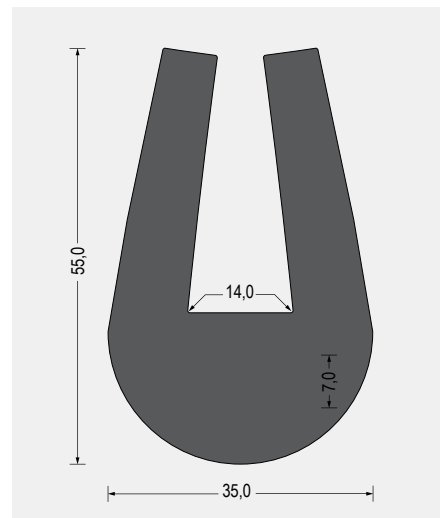
Part-Nr. 5500.1401 EPDM · 70° ShoreA · schwarz VE: Bund á 25m
