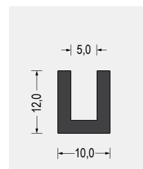
Part-Nr. 5500.0502 EPDM · 60° ShoreA schwarz VE: Bund á 100m
