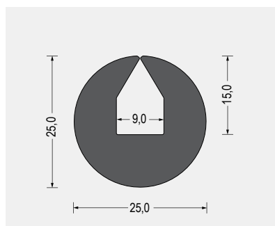
Part-Nr. 5800.6602 EPDM · schwarz VE: Bund á 25m
