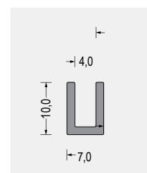
Part-Nr. 5540.0422 60° ShoreA · grau VE: Bund á 50m
