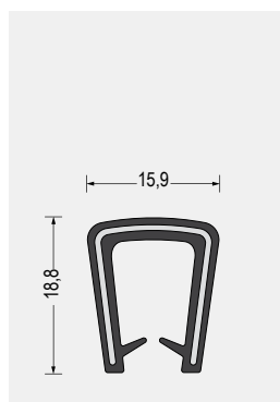
Part-Nr. 5640.8109 Silikon · schwarz Klemmbereich 6,0-10,0mm
