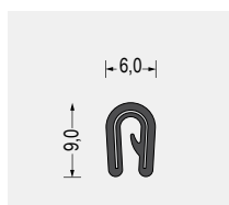
Part-Nr. 5610.0109 Soft Rubber EPDM schwarz Klemmbereich 1-2mm VE: Bund á 100m
