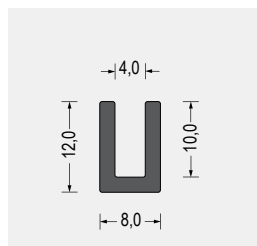
Part-Nr. 5800.6403 EPDM · schwarz VE: Bund á 50m
