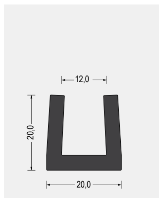
Part-Nr. 5500.1212 EPDM · 65° ShoreA · schwarz VE: Bund á 25m
