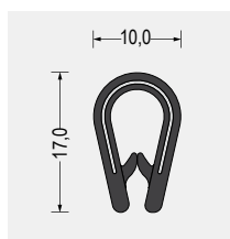
Part-Nr. 5610.1419 Weich-PVC · schwarz Klemmbereich 2-4mm VE: Bund á 100m
