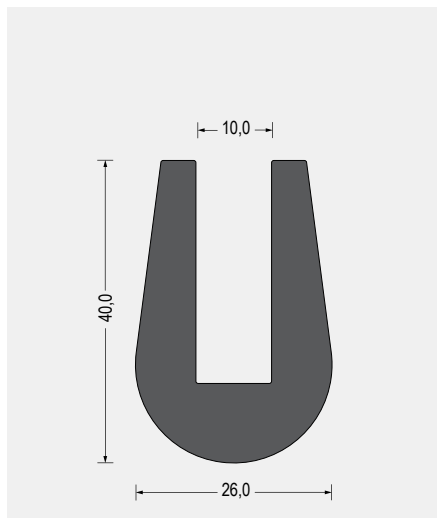
Part-Nr. 5500.1065 EPDM · 65° ShoreA · schwarz VE: Bund á 25m
