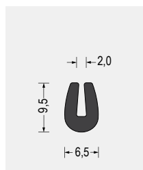
Part-Nr. 5500.0203 EPDM · 60° ShoreA schwarz VE: Bund á 100m
