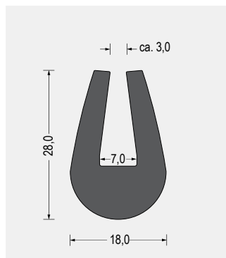
Part-Nr. 5500.0702 EPDM · 70° ShoreA · schwarz VE: Bund á 25m
