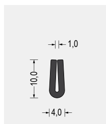
Part-Nr. 5500.0104 EPDM · 60° ShoreA schwarz VE: Bund á 200m
