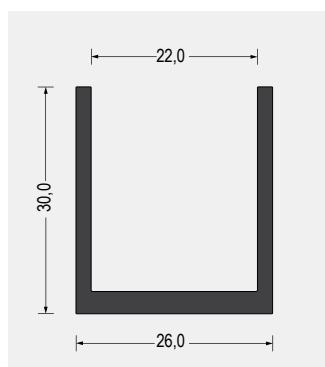
Part-Nr. 5500.2201 EPDM · 70° ShoreA · schwarz VE: Bund á 25m
