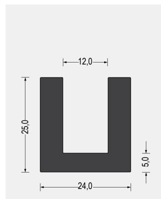
Part-Nr. 5500.1207 EPDM · 70° ShoreA · schwarz VE: Bund á 25m
