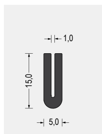
Part-Nr. 5500.0102 EPDM · 60° ShoreA schwarz VE: Bund á 100m
