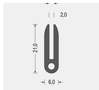
Part-Nr. 5500.0202 EPDM · 45° ShoreA · schwarz VE: Bund á 100m
