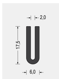
Part-Nr. 5500.0208 EPDM · 65° ShoreA schwarz VE: Bund á 50m
