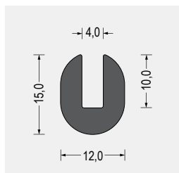
Part-Nr. 5800.7441 EPDM · schwarz VE: Bund á 50m
