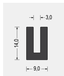
Part-Nr. 5500.0339 EPDM · 70° ShoreA schwarz VE: Bund á 50m
