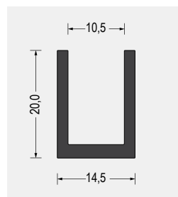
Part-Nr. 5500.1075 EPDM · 70° ShoreA schwarz VE: Bund á 50m
