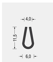
Part-Nr. 5500.0401 EPDM · 60° ShoreA schwarz VE: Bund á 100m
