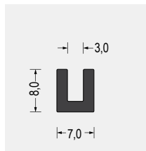
Part-Nr. 5500.0329 EPDM · 65° ShoreA schwarz VE: Bund á 100m
