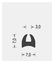
Part-Nr. 5500.0308 EPDM · 55° ShoreA schwarz VE: Bund á 200m
