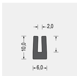
Part-Nr. 5800.6582 EPDM · schwarz VE: Bund á 100m
