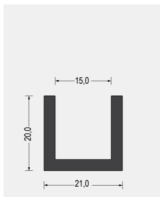
Part-Nr. 5500.1502 EPDM · 70° ShoreA · schwarz VE: Bund á 25m
