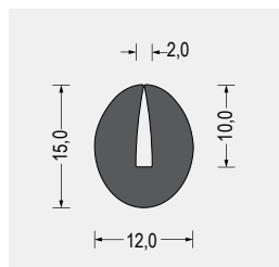
Part-Nr. 5820.5162 NBR · schwarz VE: Bund á 50m
