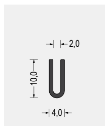
Part-Nr. 5500.0236 EPDM · 60° ShoreA schwarz VE: Bund á 100m
