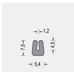
Part-Nr. 8800.7652 EPDM · grau VE: Bund á 100m
