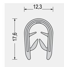
Part-Nr. 5610.1613 Weich-PVC · grau Klemmbereich 4-6mm VE: Bund á 100m
