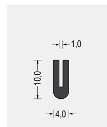
Part-Nr. 5500.0107 EPDM · 70° ShoreA schwarz VE: Bund á 50m
