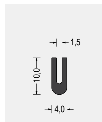
Part-Nr. 5500.0178 EPDM · 70° ShoreA schwarz VE: Bund á 100m
