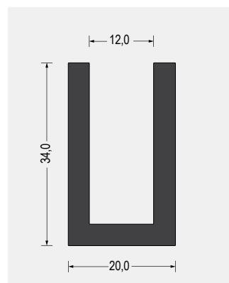
Part-Nr. 5500.1203 EPDM · 70° ShoreA · schwarz VE: Bund á 25m
