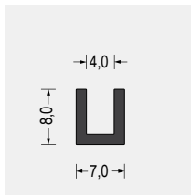
Part-Nr. 5500.0405 EPDM · 68° ShoreA schwarz VE: Bund á 100m
