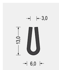
Part-Nr. 5500.0306 EPDM · 70° ShoreA schwarz VE: Bund á 100m
