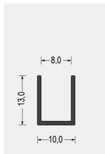
Part-Nr. 5500.0817 EPDM · 65° ShoreA schwarz VE: Bund á 100m
