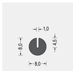
Part-Nr. 5800.5222 EPDM · schwarz VE: Bund á 50m
