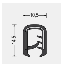
Part-Nr. 5610.1529 Weich-PVC · schwarz Klemmbereich 2-5mm VE: Bund á 100m
