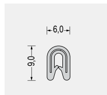
Part-Nr. 5610.1103 Weich-PVC · hellgrau Klemmbereich 1-2mm VE: Bund á 100m
