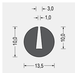
Part-Nr. 5800.9354 EPDM · schwarz VE: Bund á 50m
