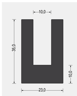
Part-Nr. 5500.1023 EPDM · 70° ShoreA · schwarz VE: Bund á 16m rundgeheizt, talkumiert
