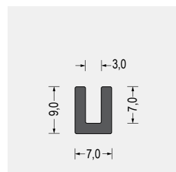
Part-Nr. 5800.6507 EPDM · schwarz VE: Bund á 50m
