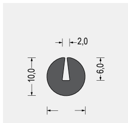
Part-Nr. 5800.5022 EPDM · schwarz VE: Bund á 50m
