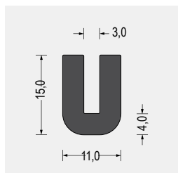
Part-Nr. 5800.5843 EPDM · schwarz VE: Bund á 50m
