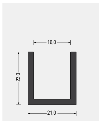
Part-Nr. 5500.1603 EPDM · 65° ShoreA · schwarz VE: Bund á 25m
