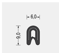
Part-Nr. 5610.1109 Weich-PVC · schwarz Klemmbereich 1-2mm VE: Bund á 100m
