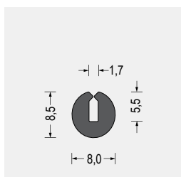
Part-Nr. 5800.6412 EPDM · schwarz VE: Bund á 200m
