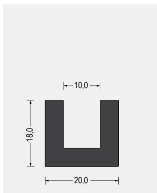
Part-Nr. 5500.1003 EPDM · 68° ShoreA · schwarz VE: Bund á 30m
