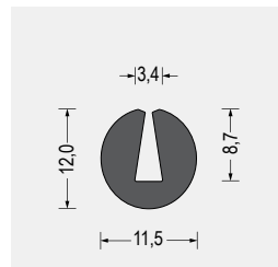
Part-Nr. 5800.5332 EPDM · schwarz VE: Bund á 50m
