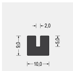
Part-Nr. 5800.7361 EPDM · schwarz VE: Bund á 50m
