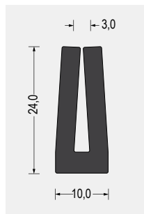
Part-Nr. 5500.0369 EPDM · 70° ShoreA schwarz VE: Bund á 15m geradegeheizt
