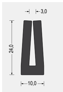
Part-Nr. 5500.0367 EPDM · 70° ShoreA schwarz VE: Bund á 15m rundgeheizt , talkumiert
