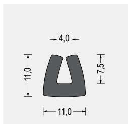
Part-Nr. 5800.5872 EPDM · schwarz VE: Bund á 50m
