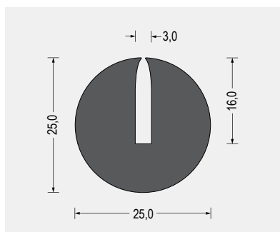
Part-Nr. 5800.9652 EPDM · schwarz VE: Bund á 25m
