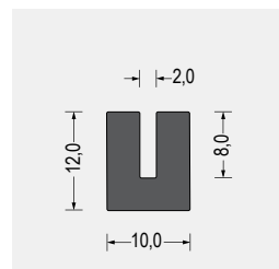
Part-Nr. 5800.5062 EPDM · schwarz VE: Bund á 50m
