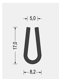
Part-Nr. 5500.0501 EPDM · 65° ShoreA schwarz VE: Bund á 100m
