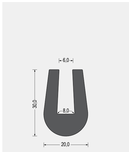
Part-Nr. 5500.0855 EPDM · 70° ShoreA · schwarz VE: Bund á 25m
