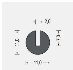
Part-Nr. 5800.5357 EPDM · schwarz VE: Bund á 50m
