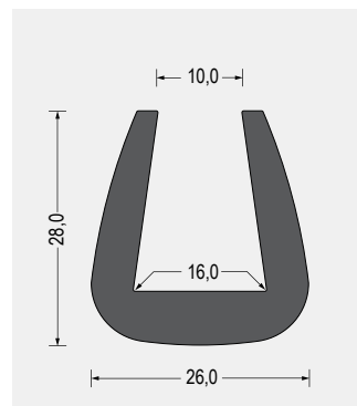
Part-Nr. 5500.1602 EPDM · 85° ShoreA · schwarz VE: Bund á 25m
