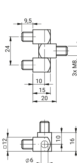
3.507.001
